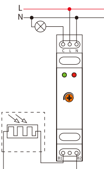
EKR8-3110系列 Working Wiring Diagram 工作接线图(SPDT)
