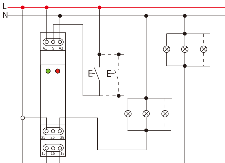
EKR8-2220 EKR8-2221 EKR8-2222 EKR8-2223系列 Working Wiring Diagram 工作接线图(DPDT)
