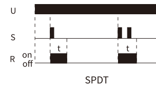
SPDT
