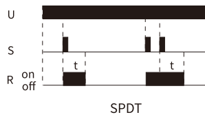
SPDT
